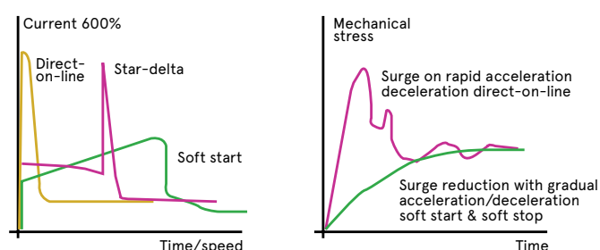
Figura 2: Curva delle prestazioni rispetto a linea diretta, Star-delta e Soft Start
